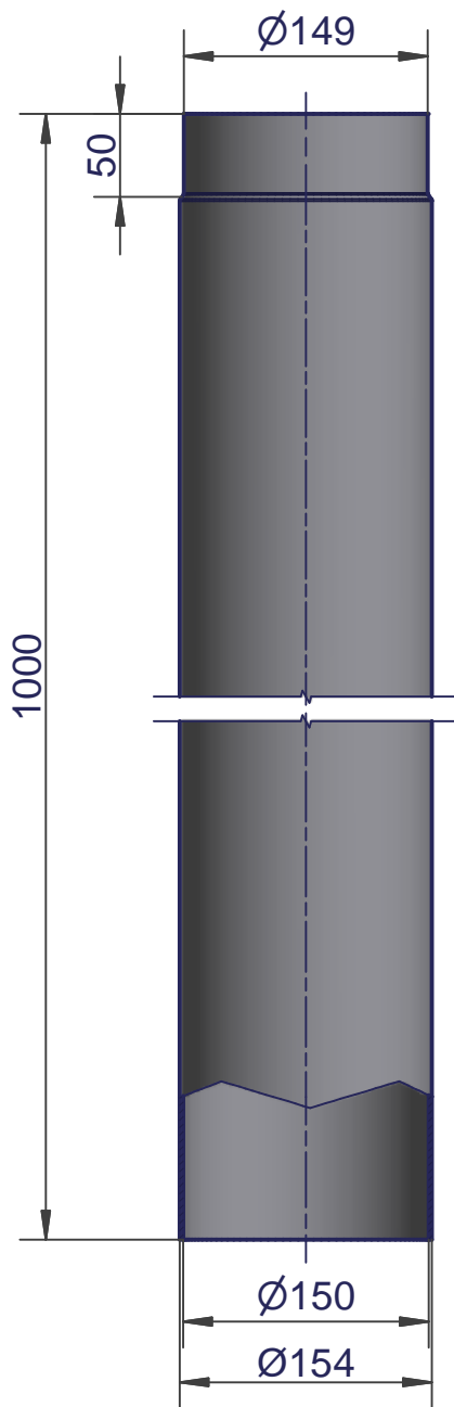
Verlängerung \text{Ø}150 \times 1000 (Maßstab 1:1)
