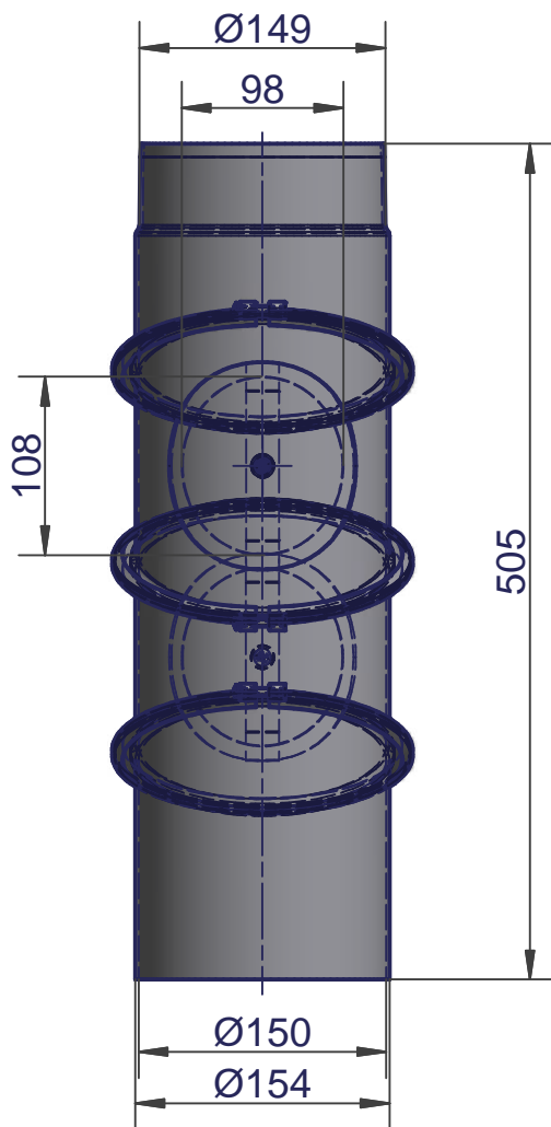
Knierohr 4 teilig verstellbar \text{Ø}150 (Maßstab 1:5)
