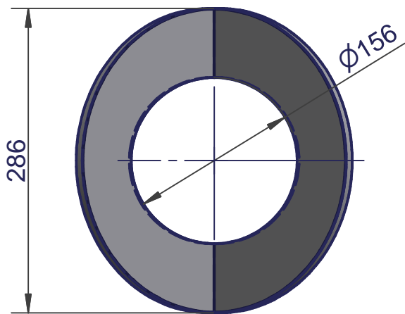
Rosette \phi 150 STD (Maßstab 1:5)
