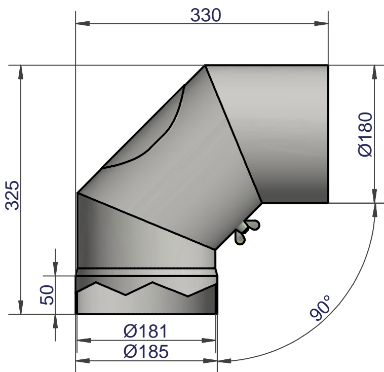
Knie STD 90°, \text{Ø}180 (Maßstab 1:5)
