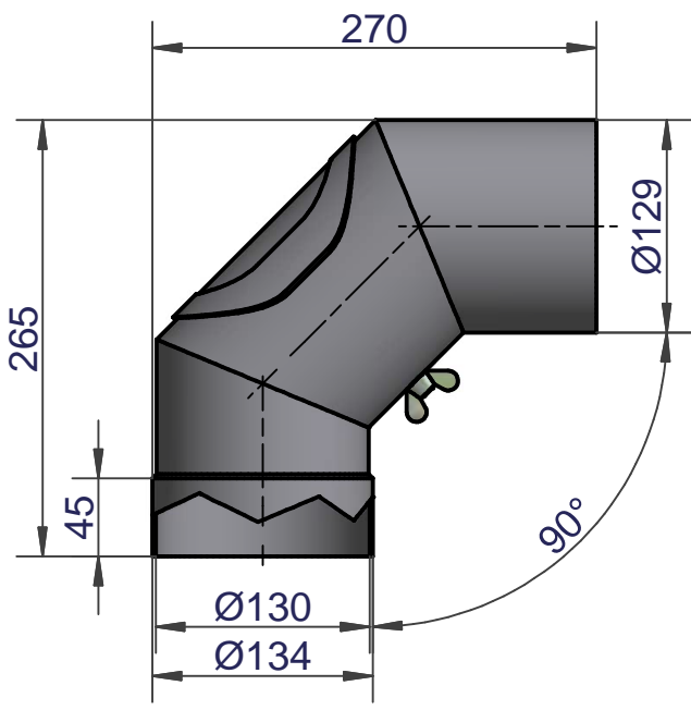
Knie STD 90°, Ø130 (Maßstab 1:5)
